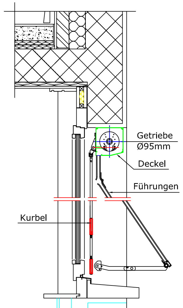
Schnitt
