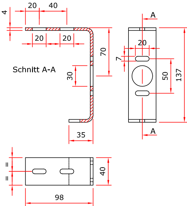
Kombilager Kabel und Alu-Stab
