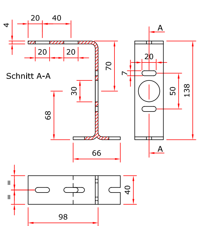
Kombilager mit Kupplung Kabel und Alu-Stab
