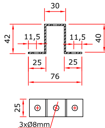
Befestigungs-Lager - nach unten -
