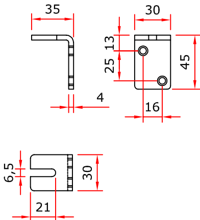
Befestigungs-Lager seitlich - unten und oben -
